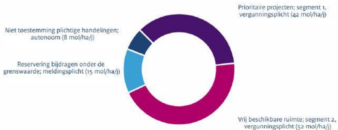
Figuur 8.1 Verdeling depositieruimte naar segment, Boschhuizerbergen (AERIUS M.2015).
