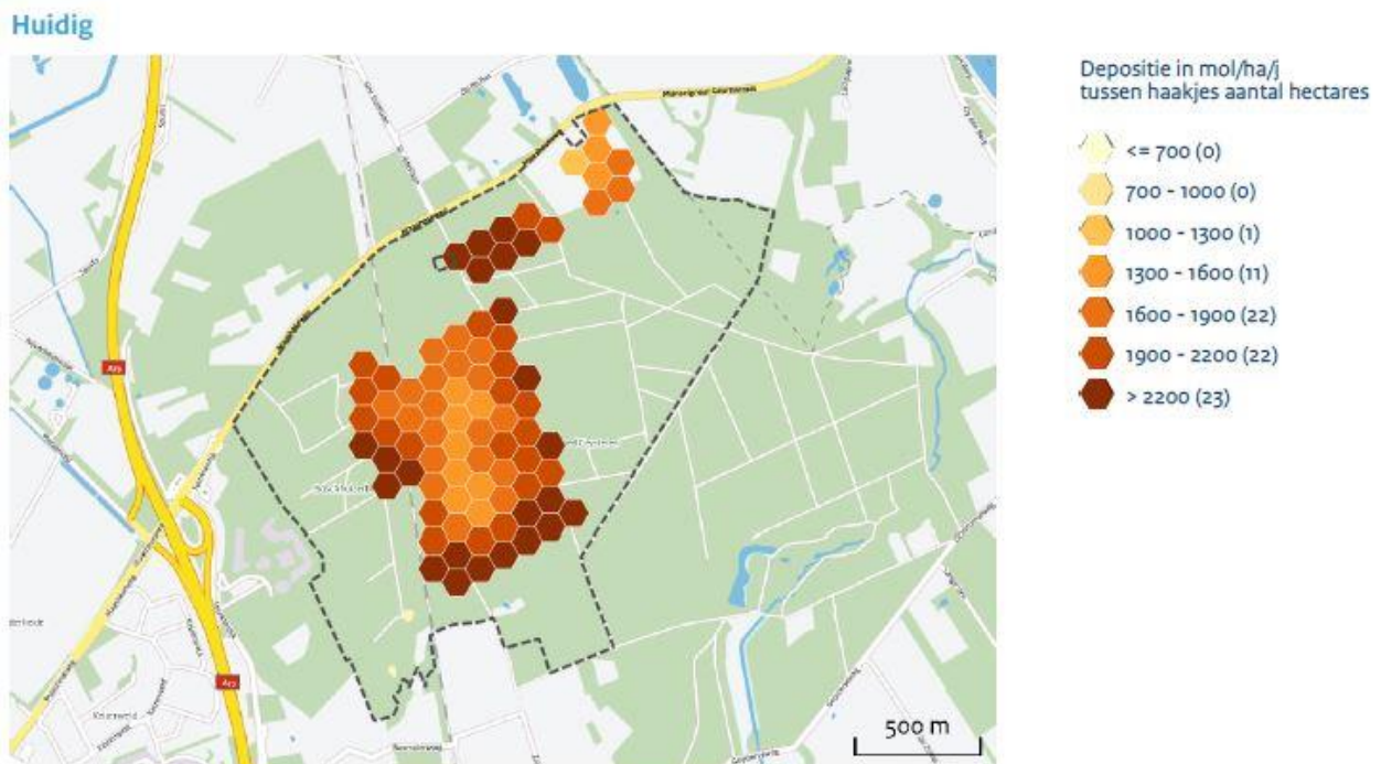
Figuur 3.2 Ruimtelijke verdeling van de stikstofdepositie per hexagoon 4 Boschhuizerbergen huidig (AERIUS M.2015).
