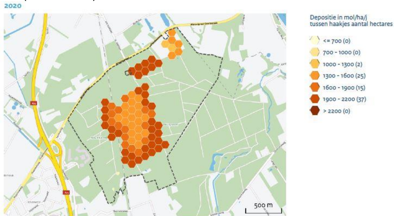
Figuur 3.3 Ruimtelijke verdeling van de stikstofdepositie per hexagoon Boschhuizerbergen 2020 (AERIUS M.2015).
