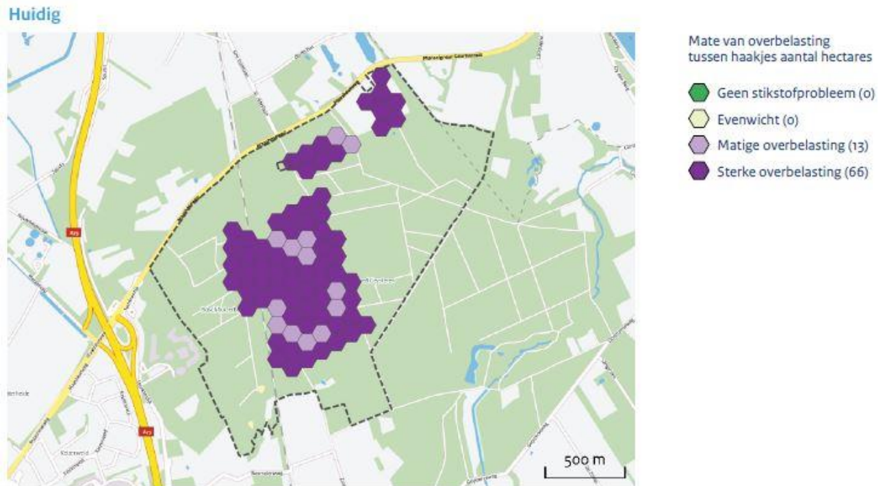
Figuur 3.5 Stikstofbelasting per hexagoon Boschhuizerbergen huidig (AERIUS M.2015).
