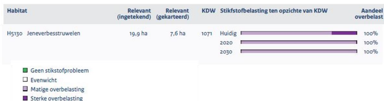
Figuur 3.11 Stikstofbelasting voor Jeneverbesstruwelen in Boschhuizerbergen (AERIUS M.2015).
