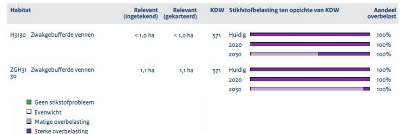
Figuur 3.10 Stikstofbelasting voor Zwakgebufferde vennen in Boschhuizerbergen (AERIUS M.2015).
