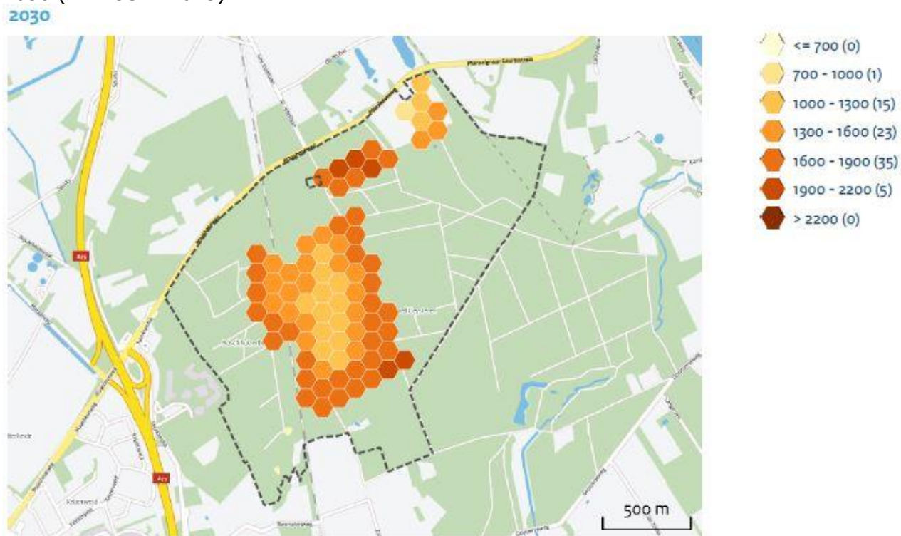
Figuur 3.4 Ruimtelijke verdeling van de stikstofdepositie per hexagoon Boschhuizerbergen 2030 (AERIUS M.2015).
