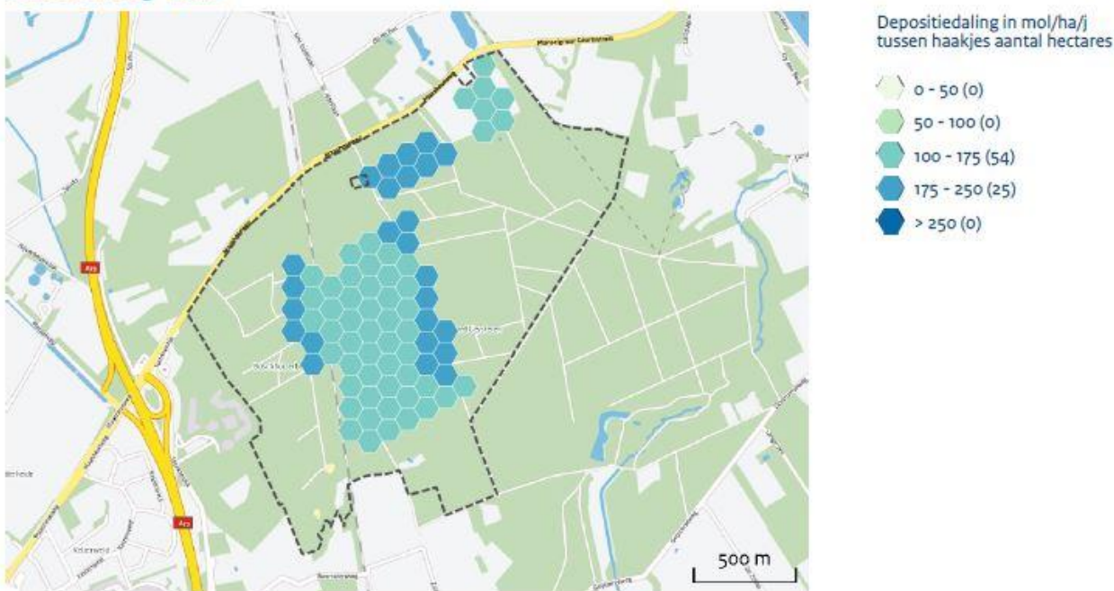
Figuur 8.2 Depositiedaling eerste PAS-tijdvak Boschhuizerbergen (AERIUS M.2015).
