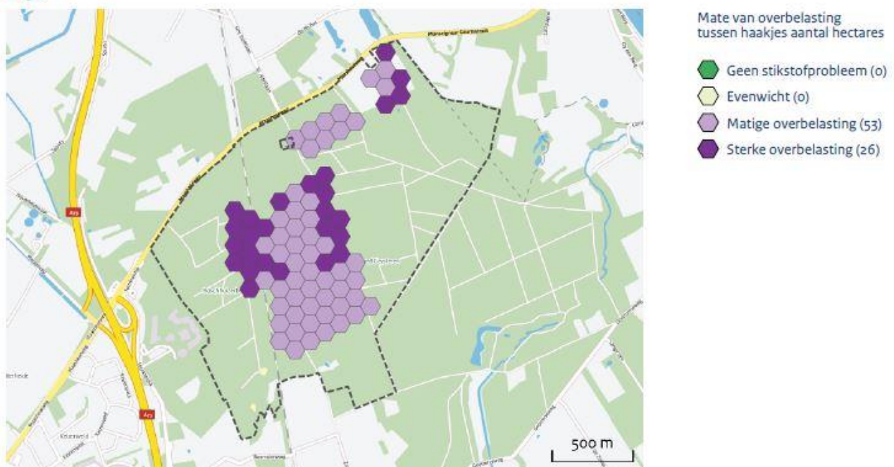
Figuur 3.7 Stikstofbelasting per hexagoon Boschhuizerbergen 2030 (AERIUS M.2015).
