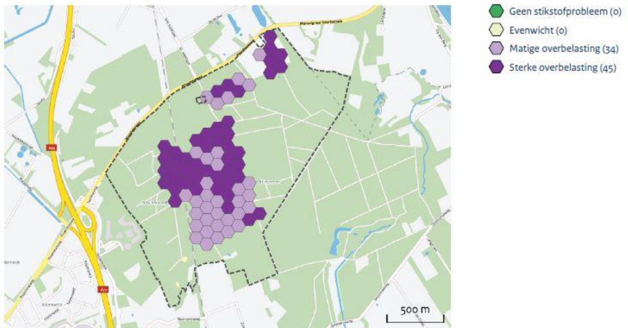
Figuur 3.7 Stikstofbelasting per hexagoon Boschhuizerbergen 2030 (AERIUS M.2015).
