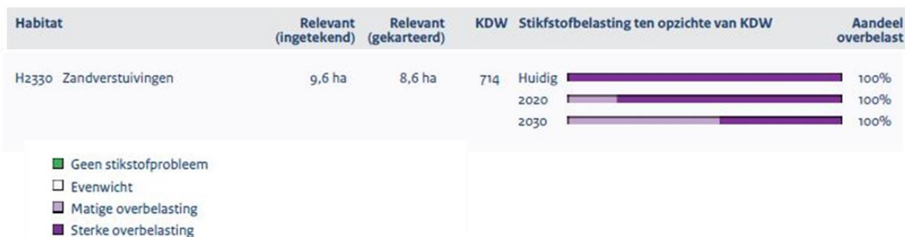
Figuur 3.9 Stikstofbelasting voor Zandverstuivingen in Boschhuizerbergen (AERIUS M.2015).
