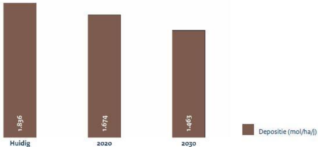
Figuur 3.1 Ontwikkeling stikstofdepositie Boschhuizerbergen (AERIUS M.2015).
